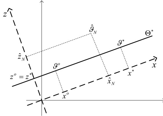
Figure 1. The parameter space
